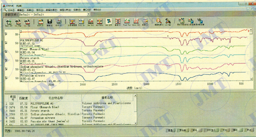
PP 塑料样品红外谱图与聚丙烯标准红外谱图的匹配图
